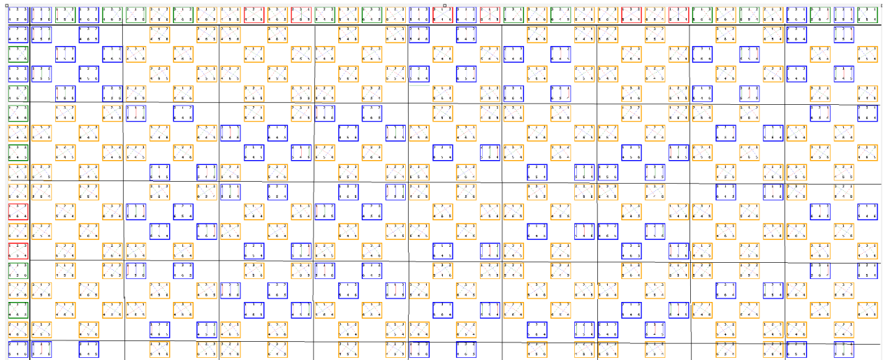
ELECTROMAGNETISMUL CU COMPONENTA ELECTRICĂ (GALBEN) SI MAGNETICĂ (ALBASTRU)
